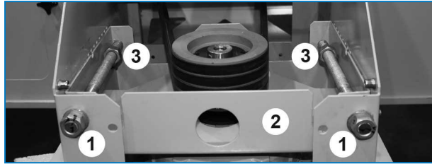
Base motore regolabile
