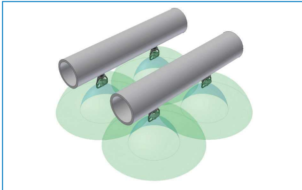
Tipo distribuzione spruzzi dagli ugelli per torre di raffreddamento a circuito chiuso
