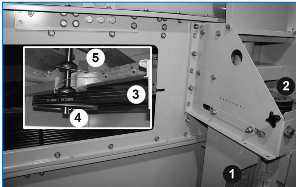
Sistema di azionamento con motore esterno
