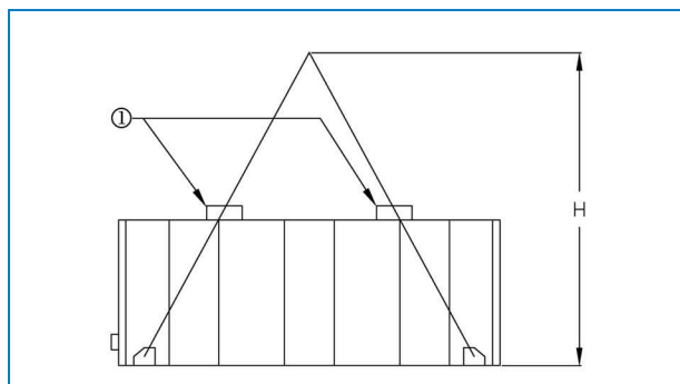
1. Spreidingsbalk
