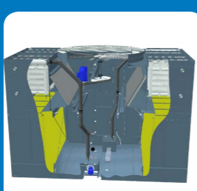
Esecuzione per alte temperature CPVC BACross 2 pacco di scambio
