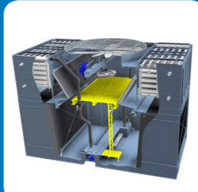
Piattaforma interna con scala
